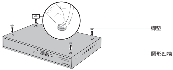
图2-1 桌面安装示意图
