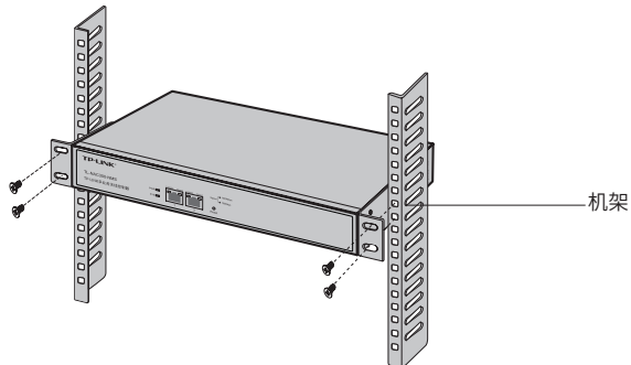
图2-3 机架安装示意图
