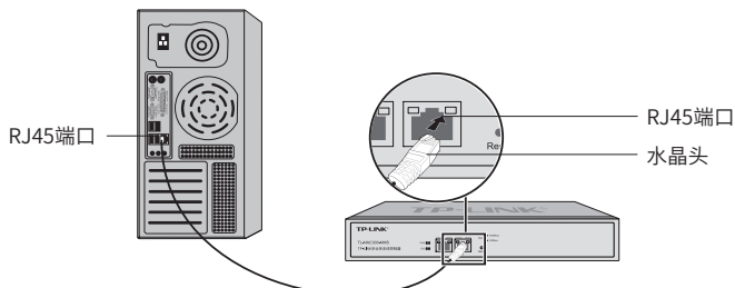
图3-1 无线控制器连接线缆示意图
